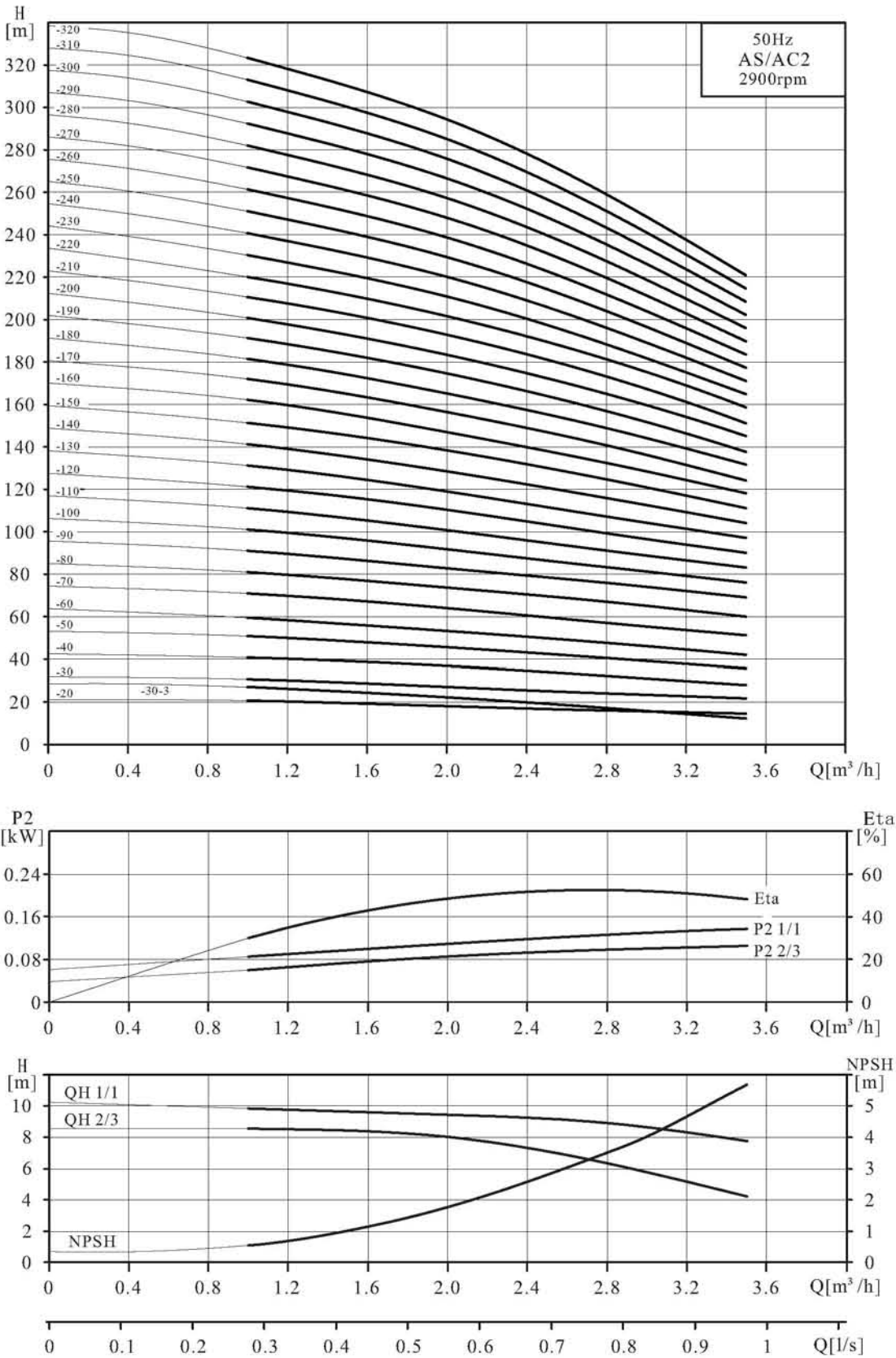
性能曲线
